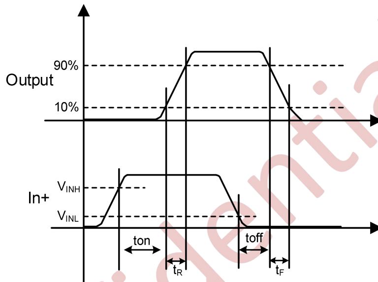
图 8-1 输入输出（同相）波形图
