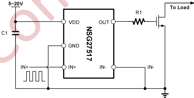
图 9-2 NSG27517 同相典型应用电路图
