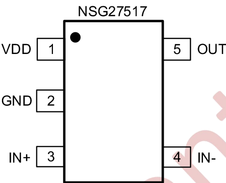
图 6-1 5 脚 SOT23-5 顶视图
