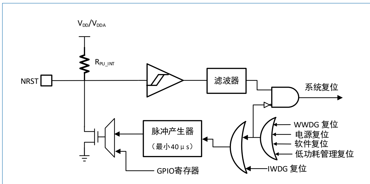
图 3-3 复位信号
