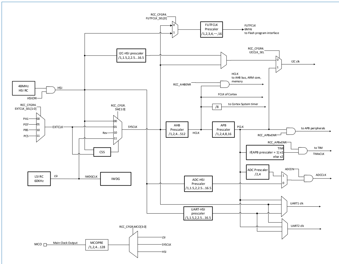
图 3-4 HK32G003 时钟树
