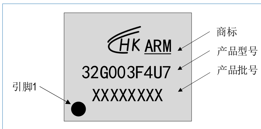
图 7-10 QFN20 HK32G003F4U7 丝印示例
