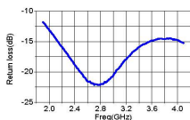
典型特性曲线
