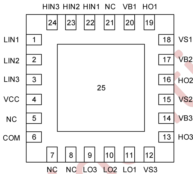
图 7-1 NSG6288Q QFN24 顶视图
