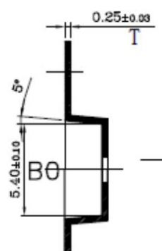
B-B
