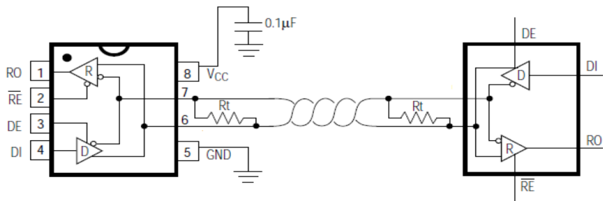
图 1: SN75LBC184DR-TD典型半双工应用电路
