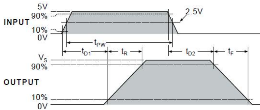
图 9-2 输入输出(B 通道同相) 波形图
