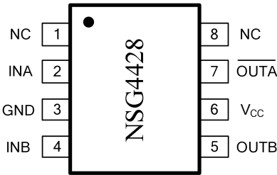
图 7-1 8-脚 SOP8 顶视图
