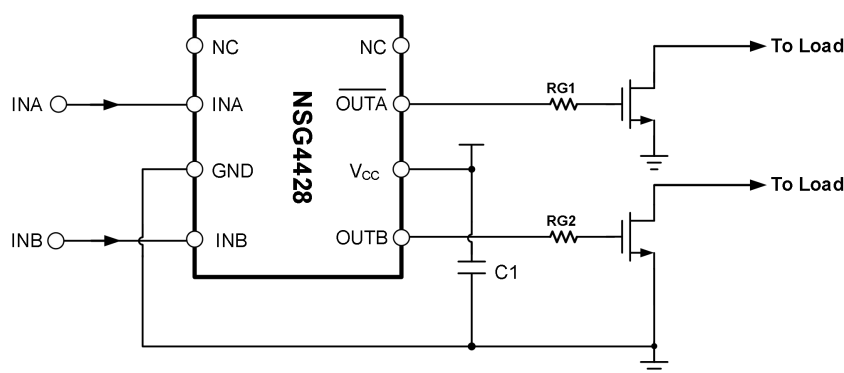
图 11-1 NSG4428 典型应用电路图
