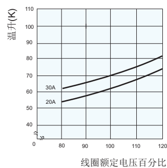
线圈温升
