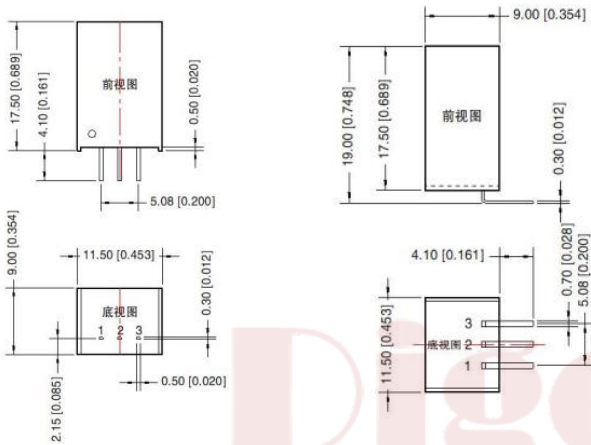
图3：外型尺寸
