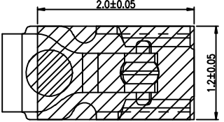
焊盘尺寸
