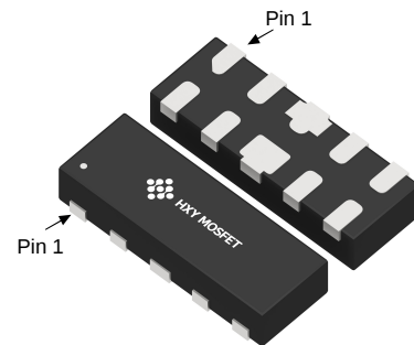
DFN2510-10L (UFDN-10)
