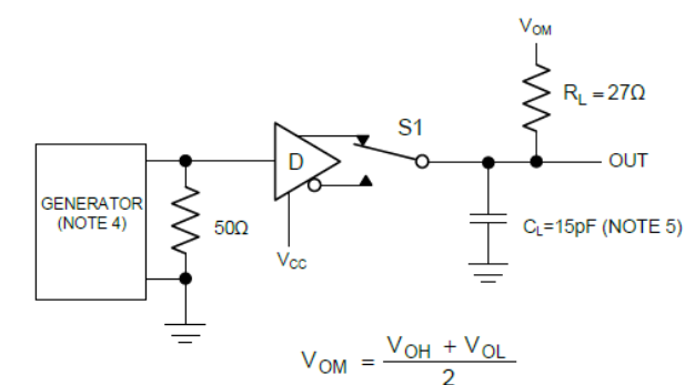
图 1 发送 V_{OD} 和 V_{OC}
