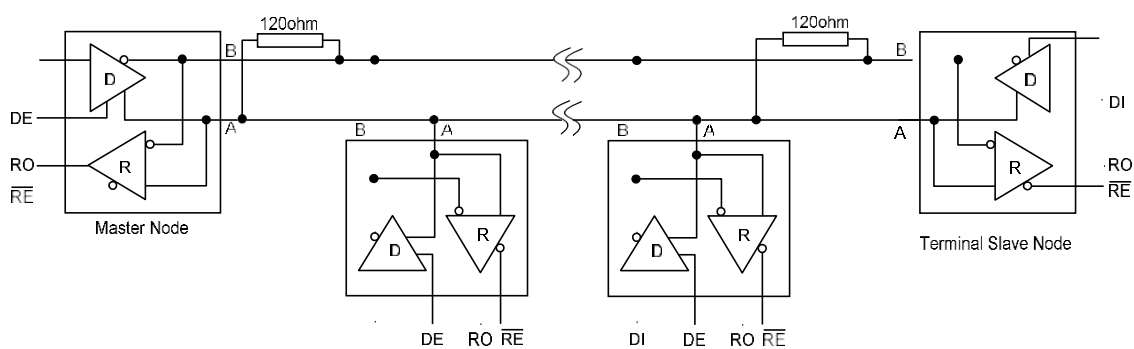
图 9 典型半双工 RS-485 组网应用
