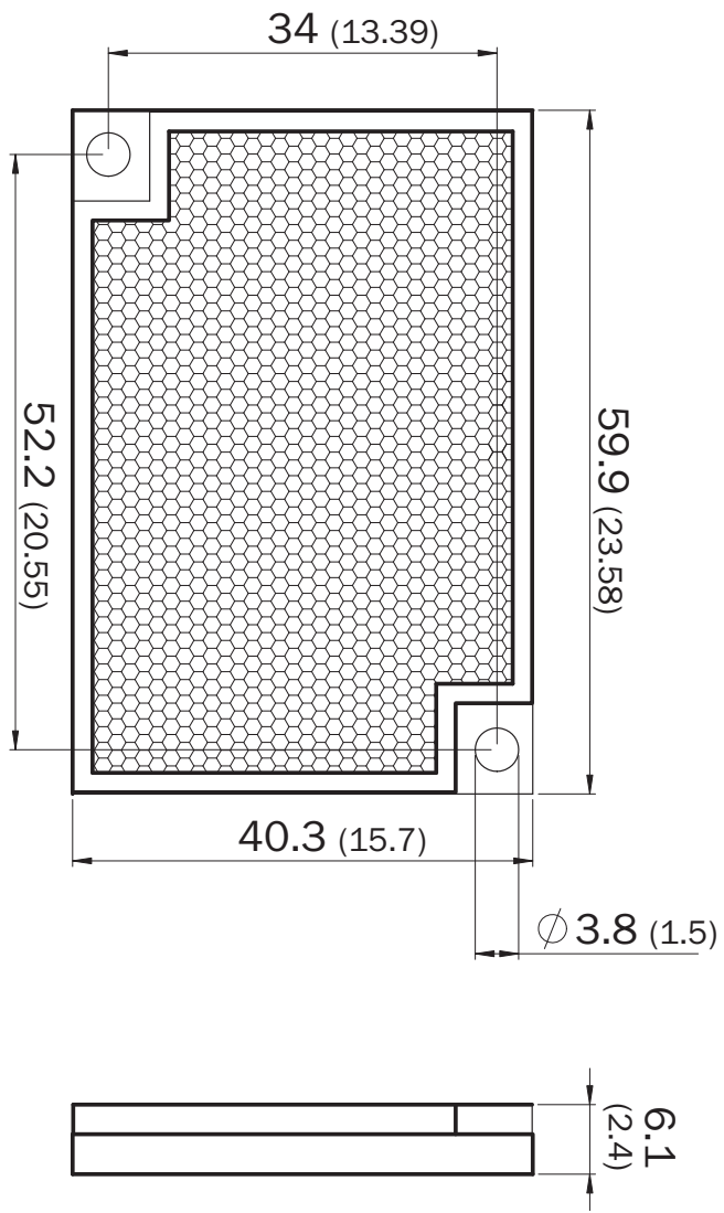
尺寸图 (尺寸单位: mm)
