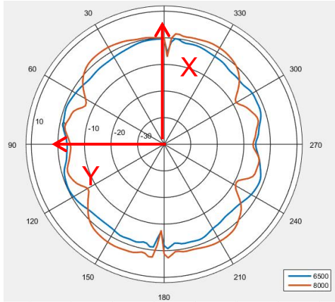
2D-theta=90
