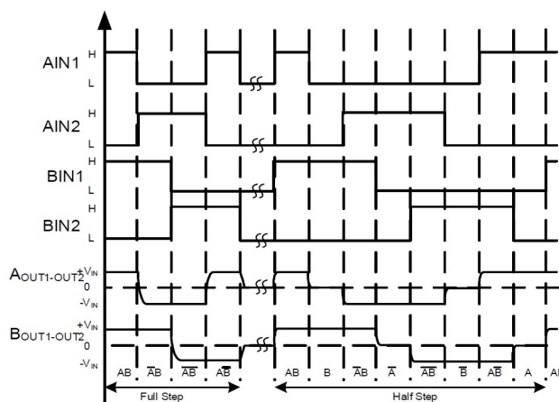
图 5 全步和半步的信号逻辑序列
