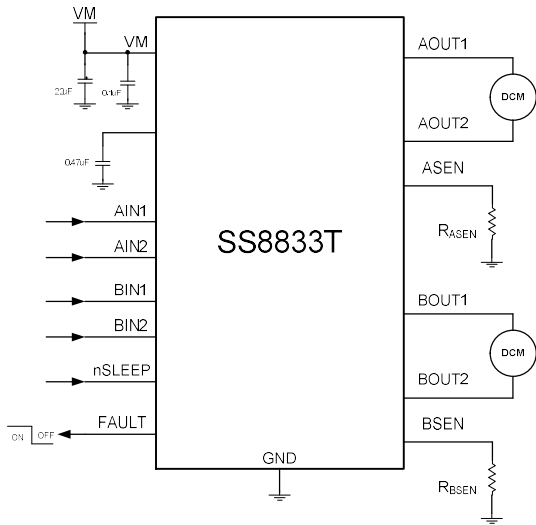
双直流电动机的应用
