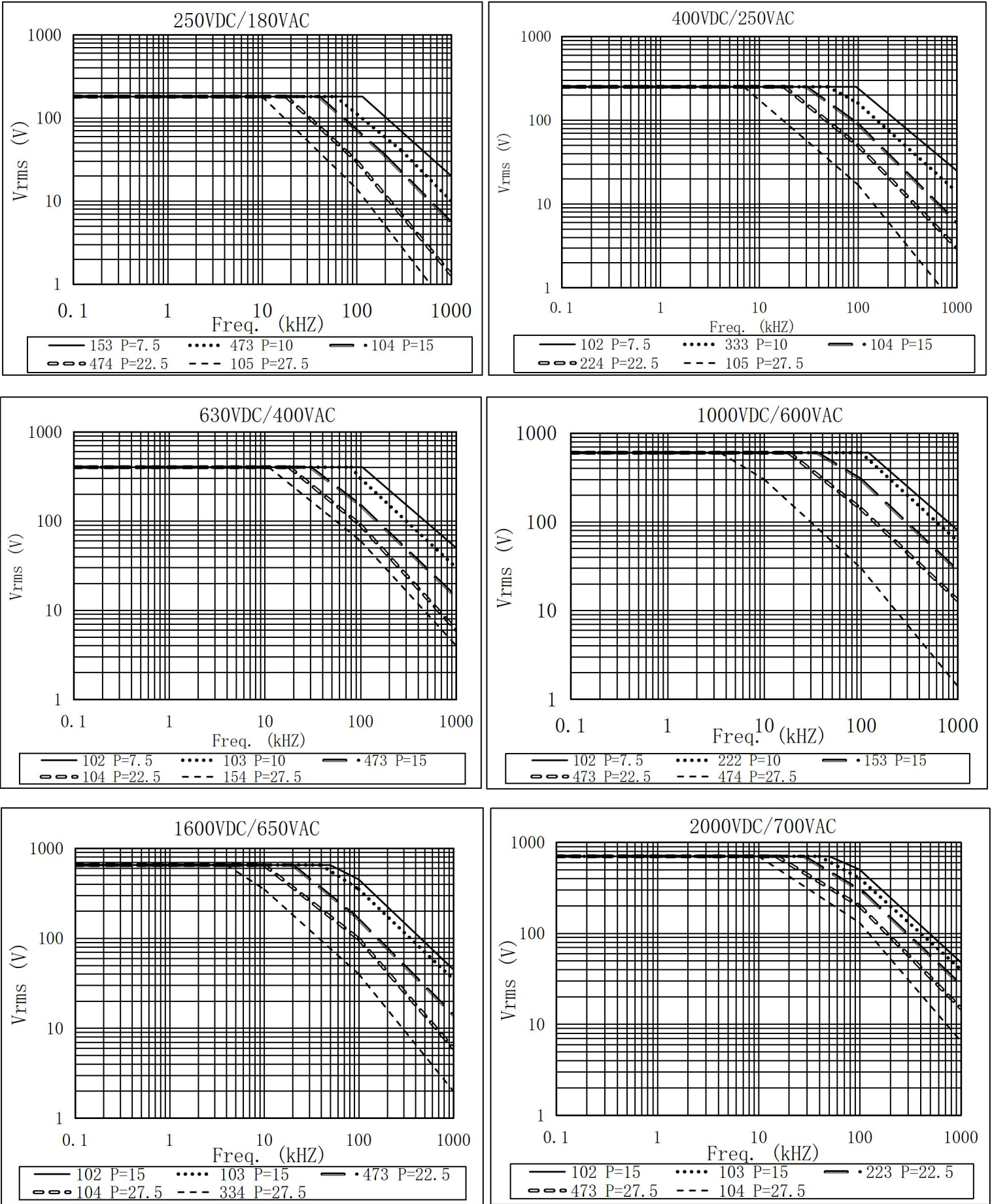
最大可允许电压（Vr.m.s）——频率特性曲线
