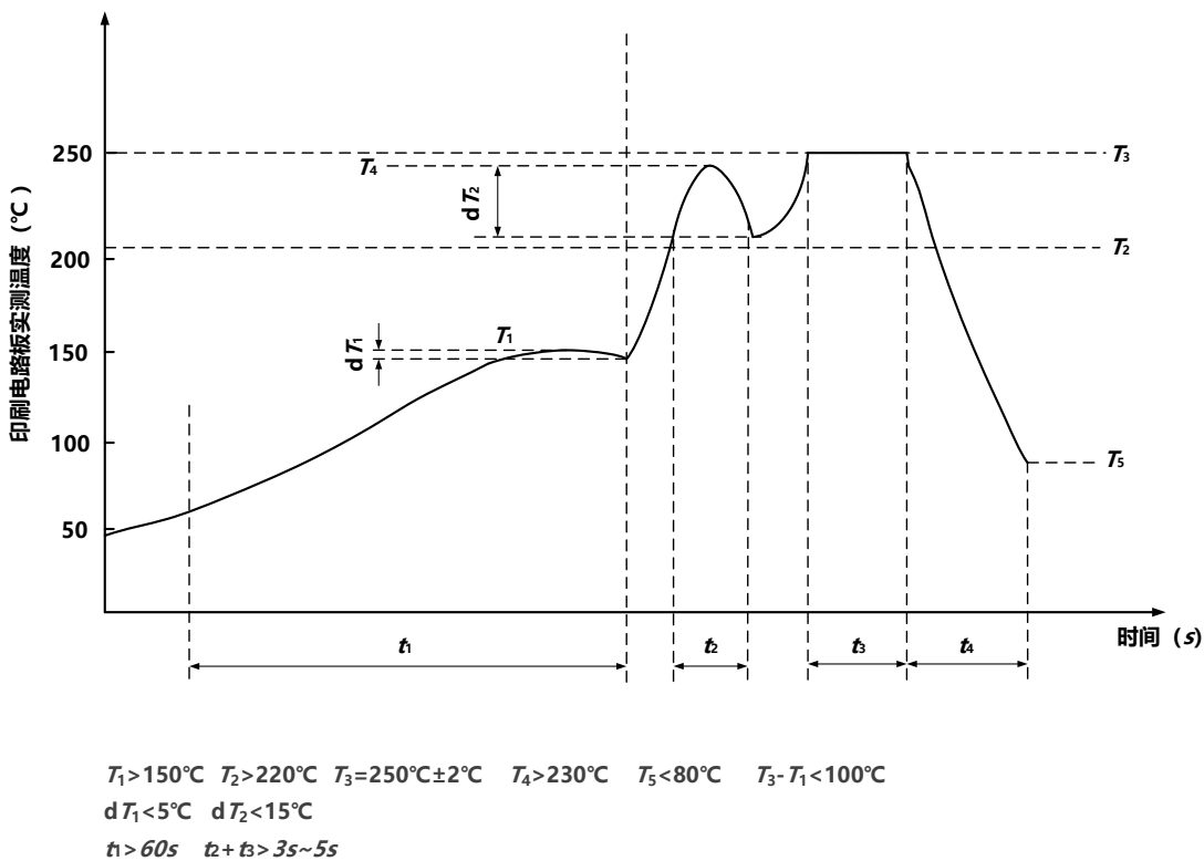
图 7 无铅波峰焊接温度曲线推荐图
