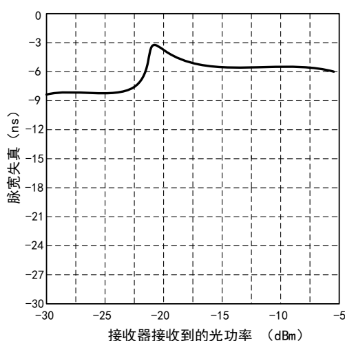
图2 在 5MBd 速率下 NRS15x1ETZ/25x1ETZ 的脉宽失真
