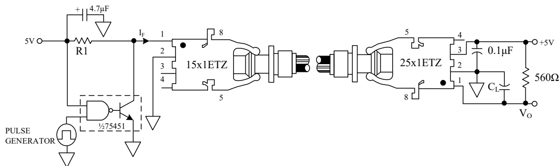
图 4 NRS15x1ETZ/25x1ETZ 典型应用电路图
