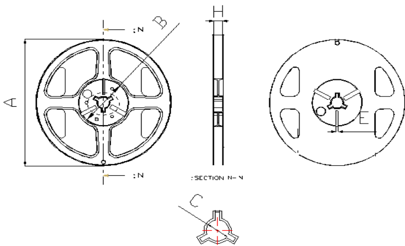
图3 圆盘 表8 圆盘尺寸
