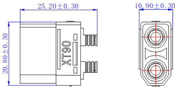
带后盖堆叠尺寸
