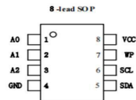
SOIC-8
