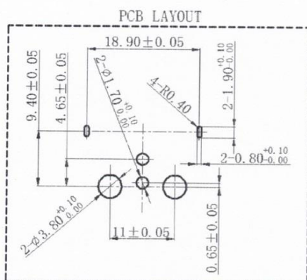
PCB 安装孔示意图
