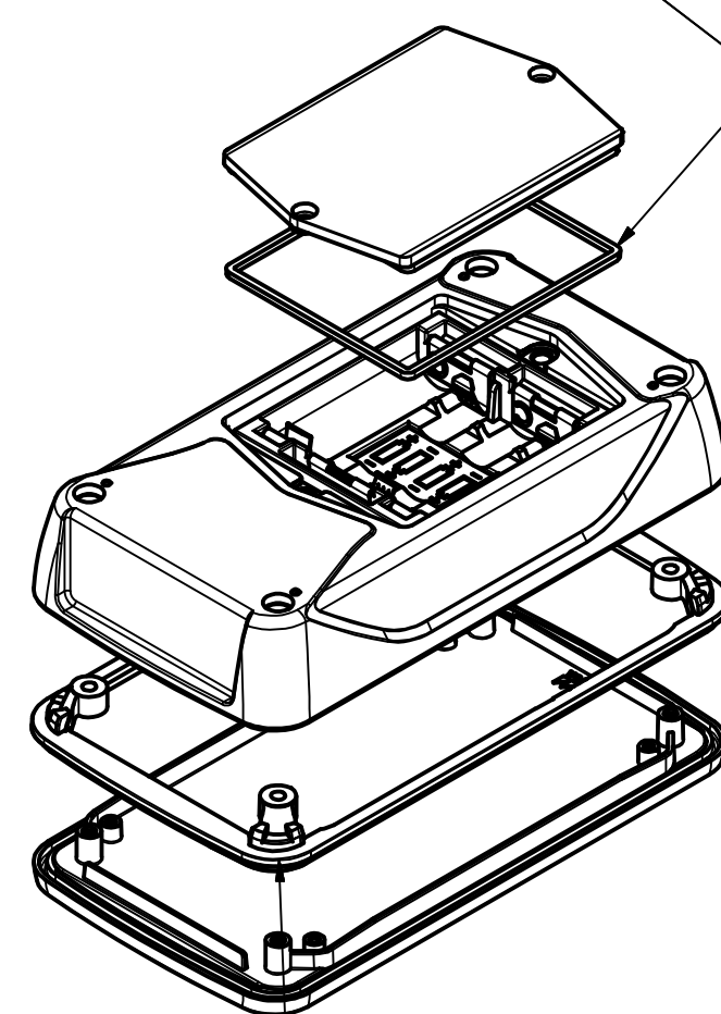
Gehäusedichtung Enclosure seal
