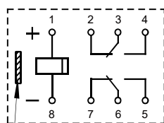
单稳态
