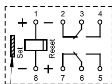
单线圈磁保持
