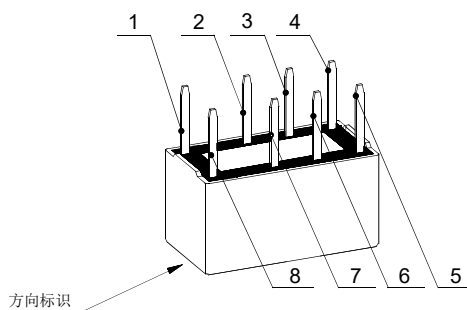
脚位示意图
