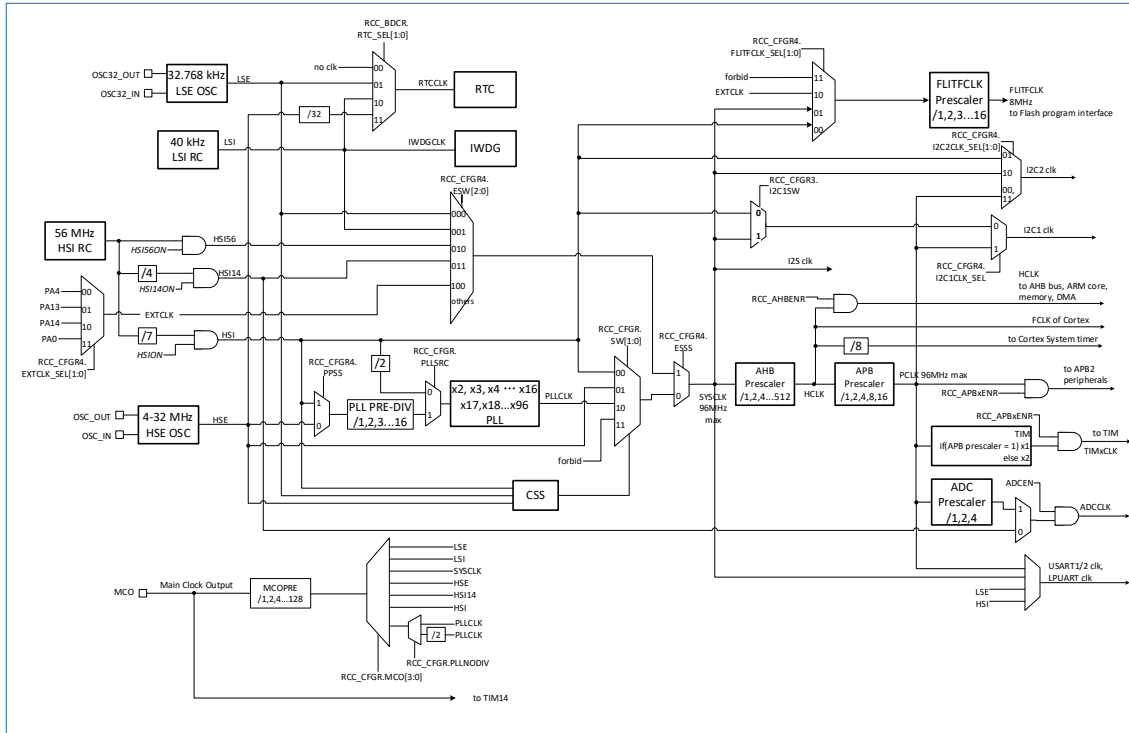
图 3-4 HK32F030xxxxA 时钟树
