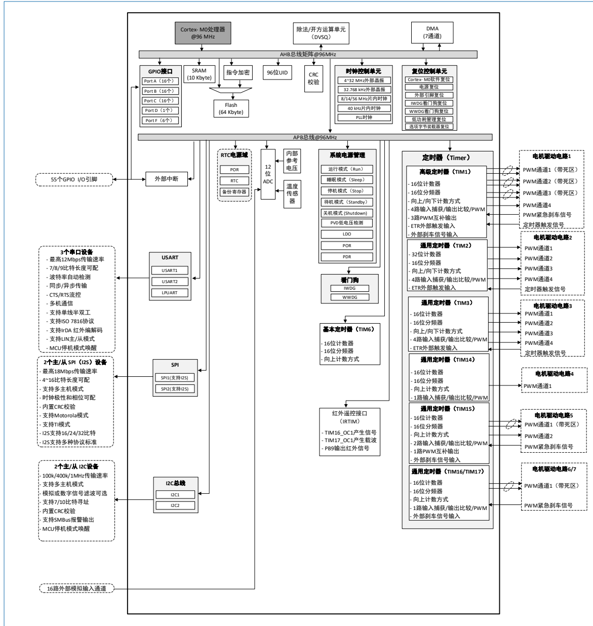
图 3-1 HK32F030R8T6A 功能框图
