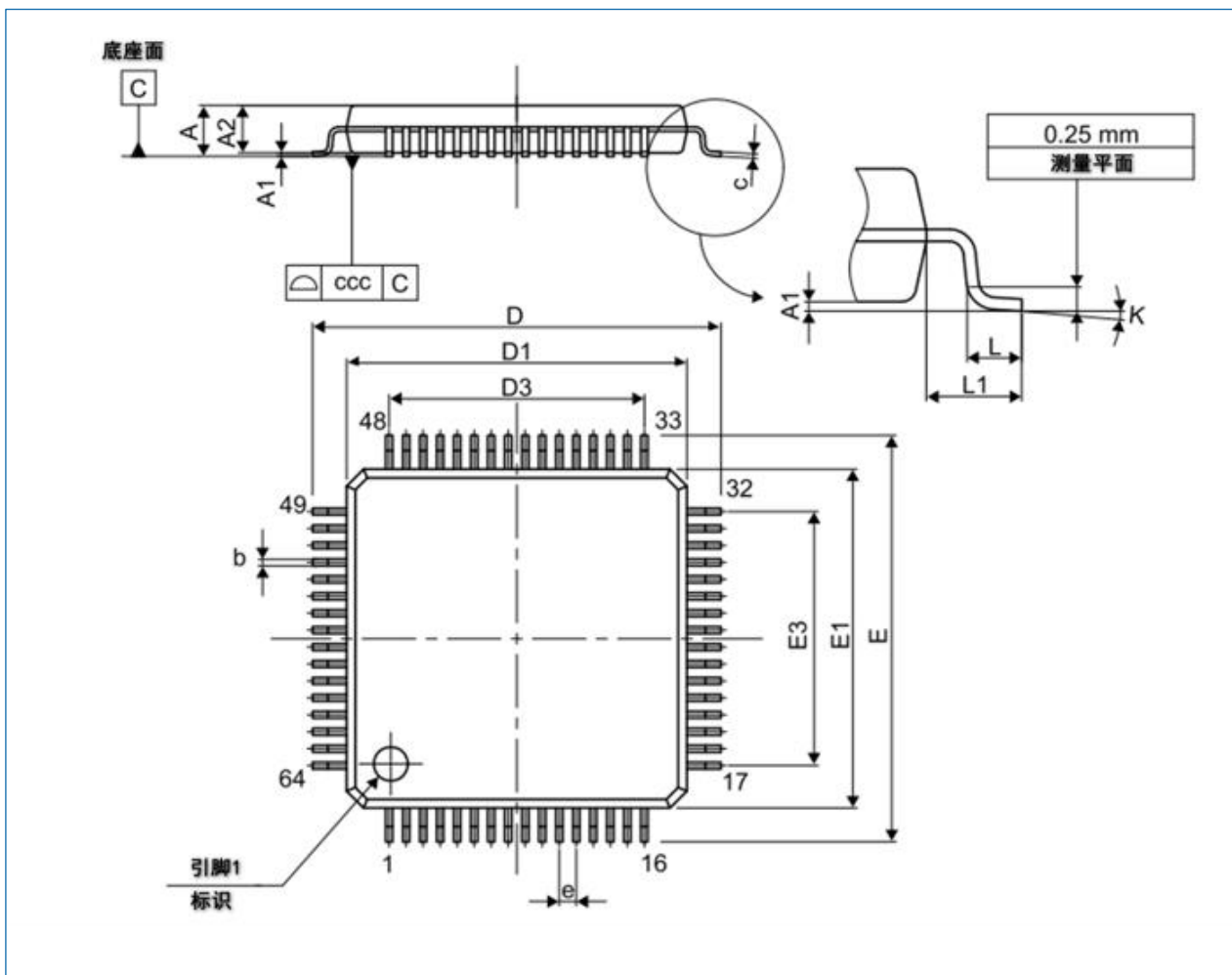
图 7-1 LQFP64 封装尺寸图
