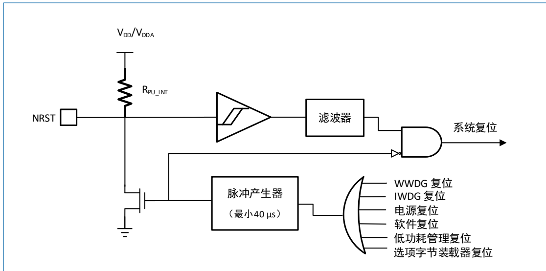
图 3-3 复位信号
