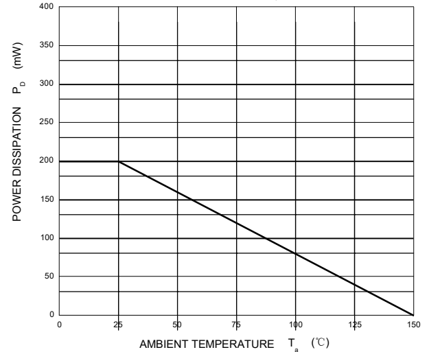
P_D — T_a
