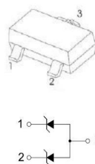
SOT-23
