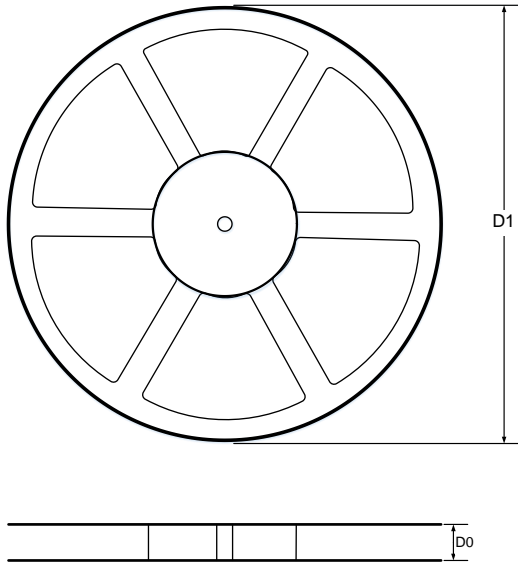
REEL DIMENSIONS
