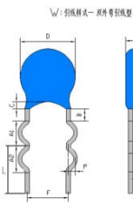
双外弯引线型
