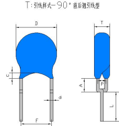
90°前后翘脚型引线
