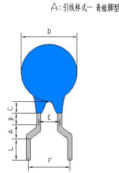
青蛙脚型引线
