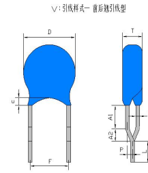
前后翘脚型引线
