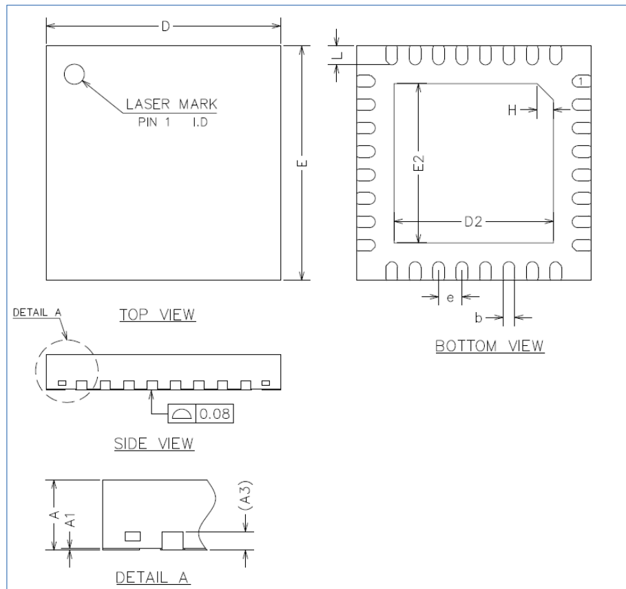
图 7-5 QFN32 封装尺寸
