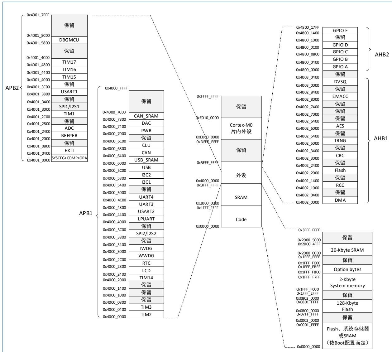
图 3-2 HK32L088RBT6 存储器映射
