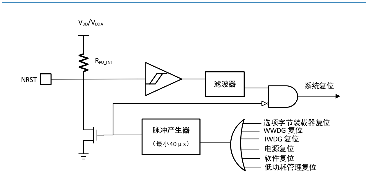
图 3-3 复位信号
