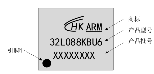
图 7-14 QFN32 HK32L088KBU6 丝印示例
