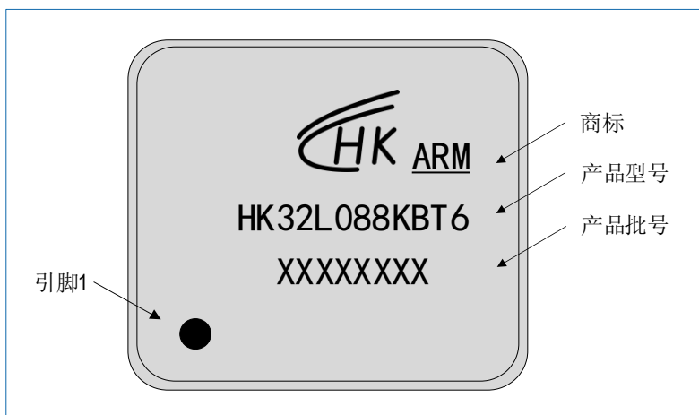
图 7-11 LQFP32 HK32L088KBT6 丝印示例
