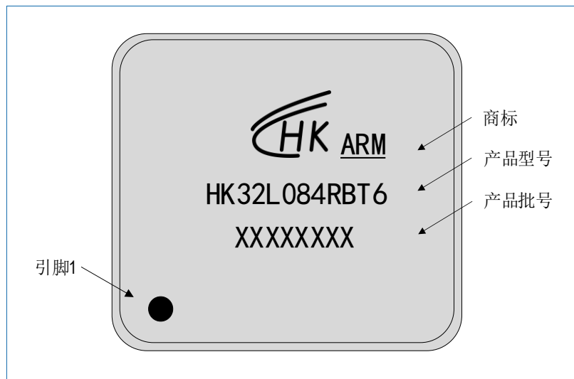
图 7-6 LQFP64 HK32L084RBT6 丝印示例
