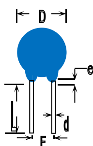
TYPE A: 直脚 Straight
