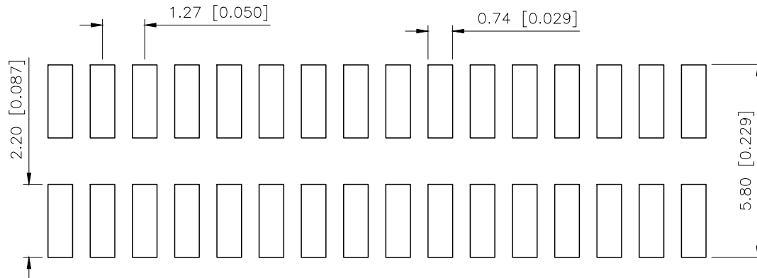
P.C.B LAYOUT
