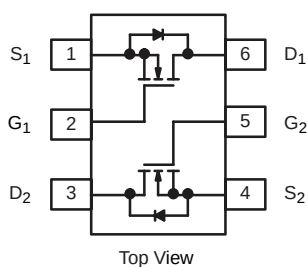
SOT-363 SC-70
