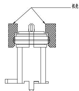
组装示意图
