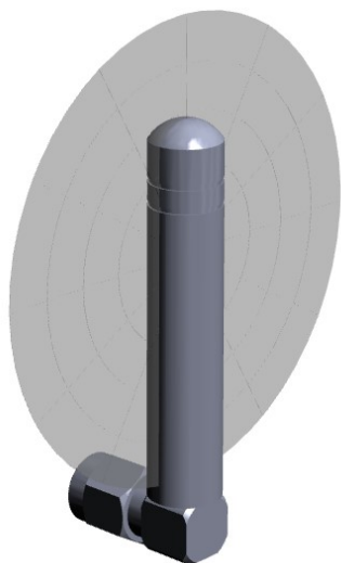
XZ-Plane Gain
