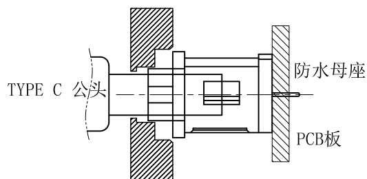
组装示意图
