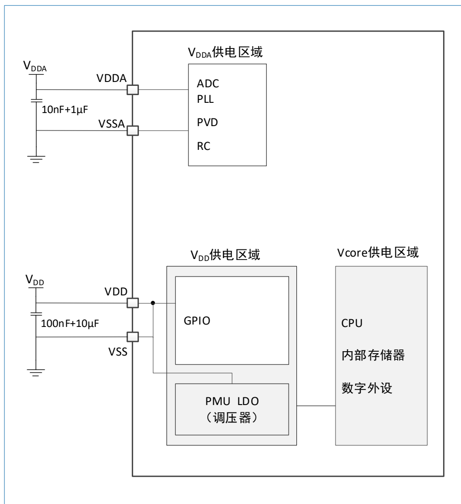
图 5-1 电源框图
