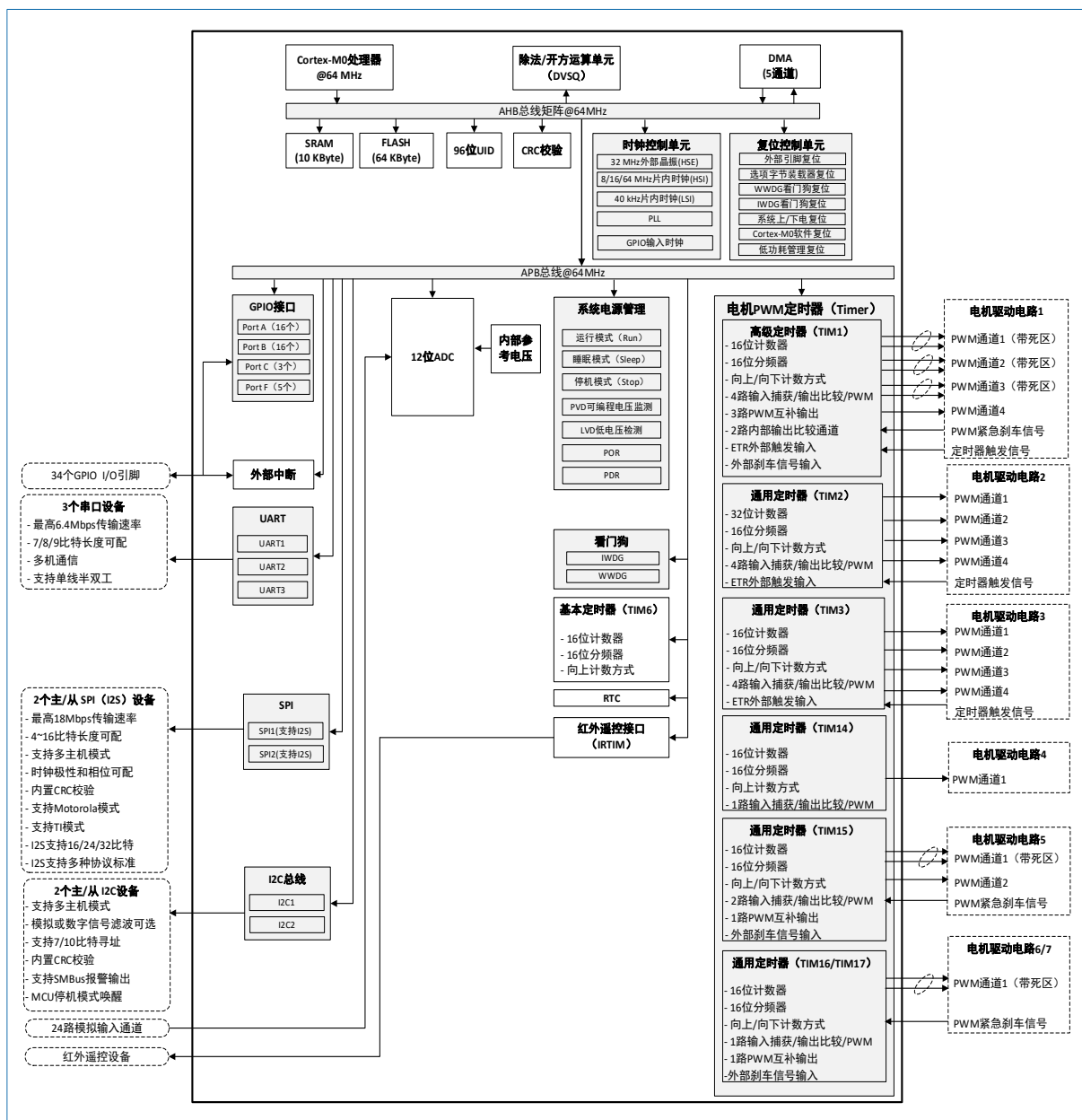
图 3-1 HK32C207S8T7 功能框图
