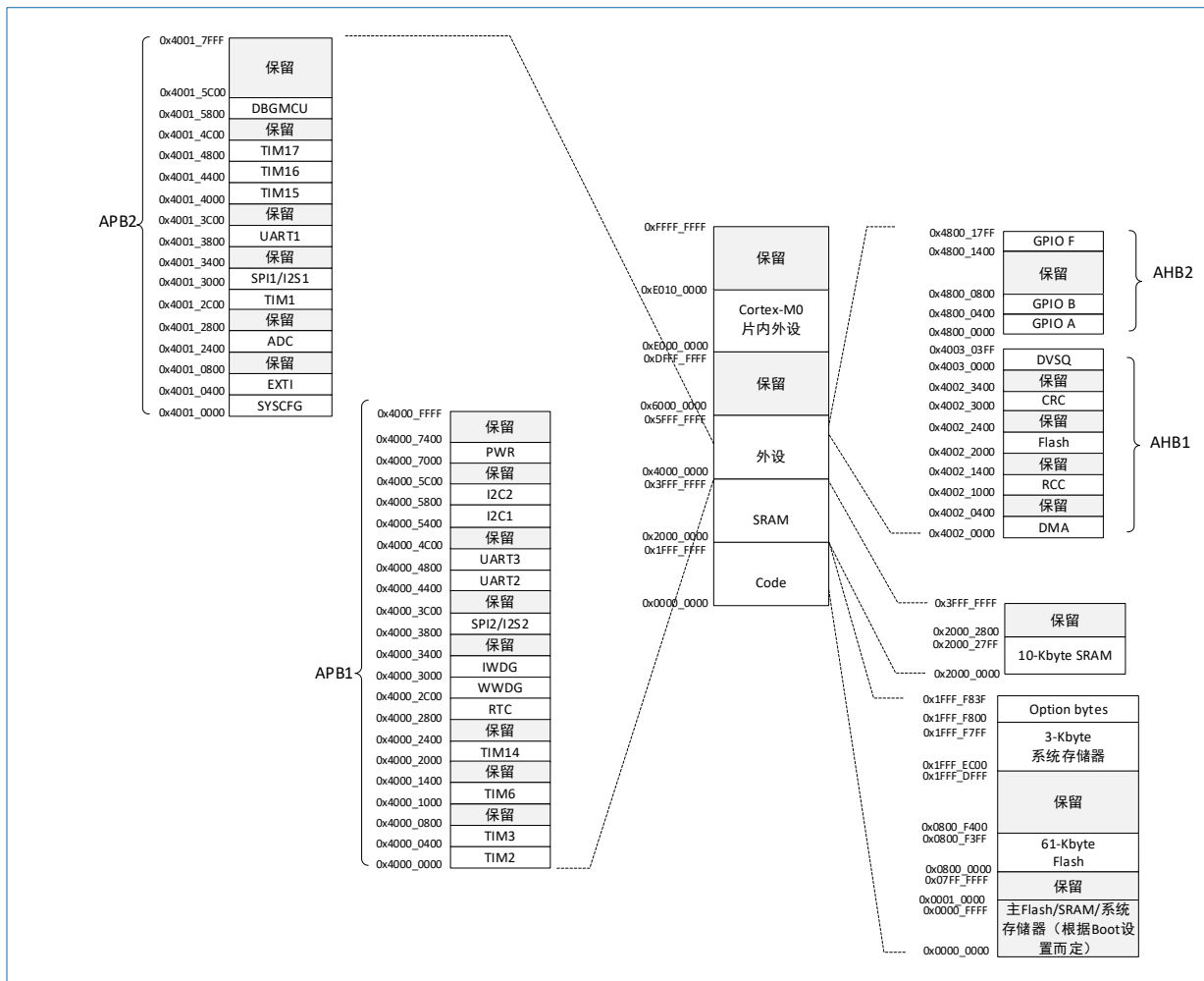
图 3-2 HK32C207 存储器映射
