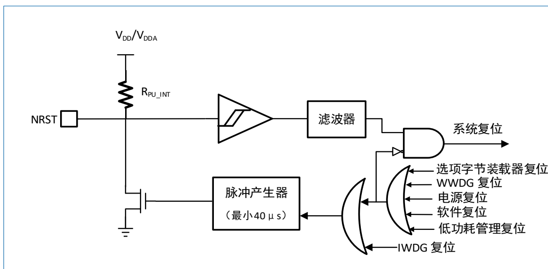
图 3-3 复位信号
