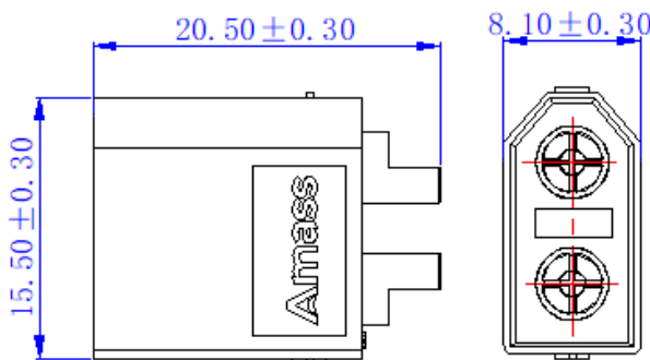
堆叠尺寸
