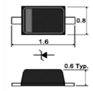
SOD-523F Unit:mm
