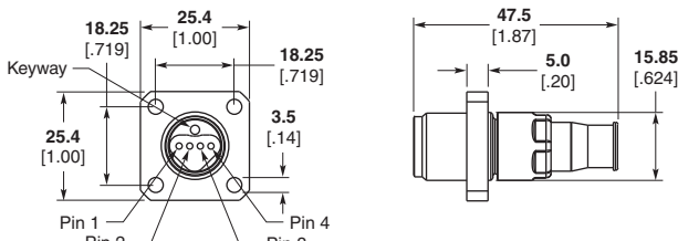
ODC 4 Fiber Socket Small Square to LC
