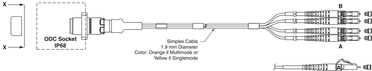
ODC 4 Fiber Socket Small Square to LC
