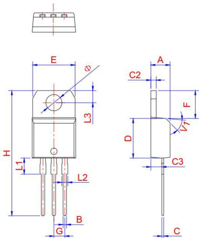
TO-220A Ins
