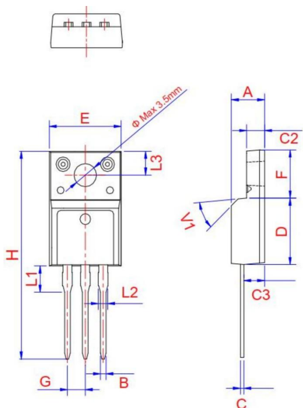
TO-220F Ins
