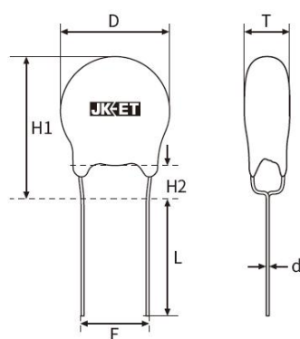
类型 D：Y 形脚
