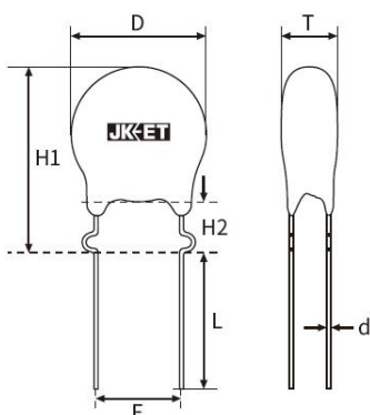
类型 C：外 K 脚
