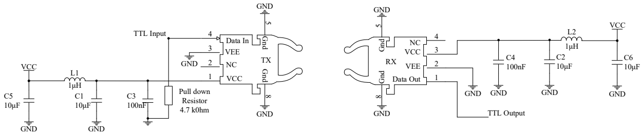
图 1 NRS16xxZ/26x4Z/25x9Z 典型应用电路图
