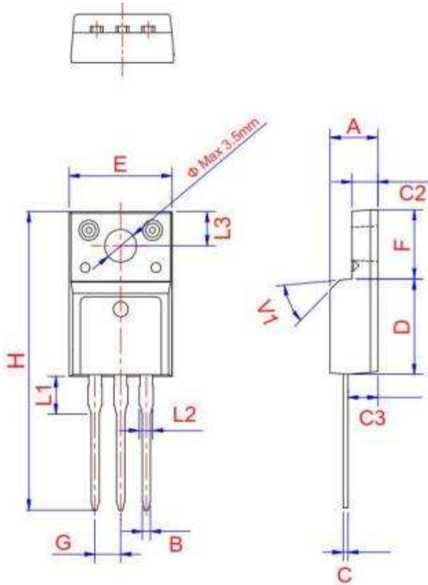
TO-220F Ins
