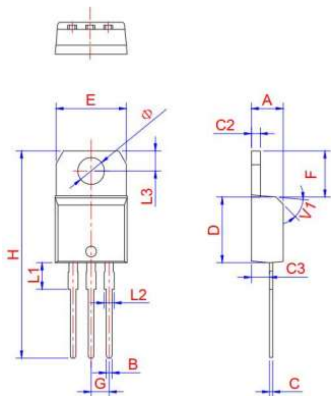
TO-220A Ins
