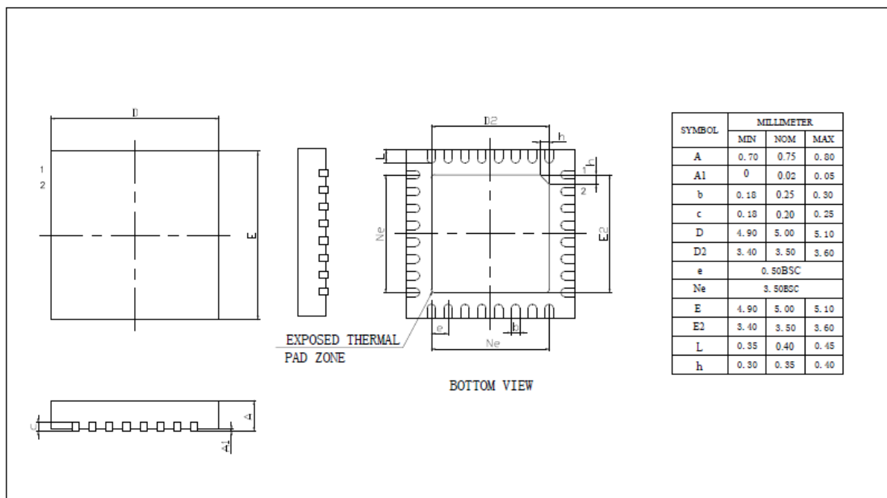
图 5-2 QFN32(5mmx5mm)封装尺寸
