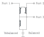
原理框图
