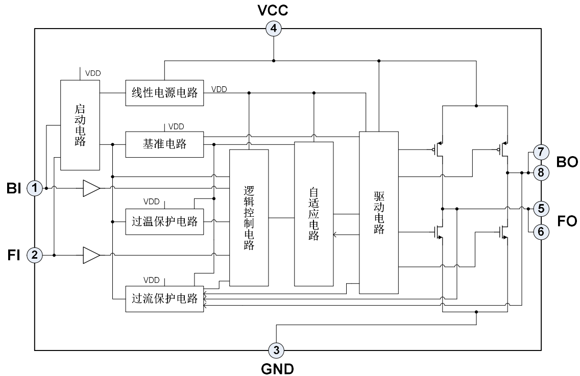
图 3. 主要模块框图
