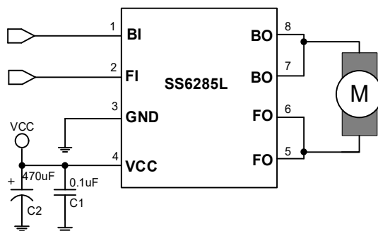
图 4. 应用原理图
