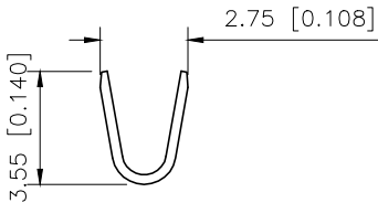
SEC:B-B
