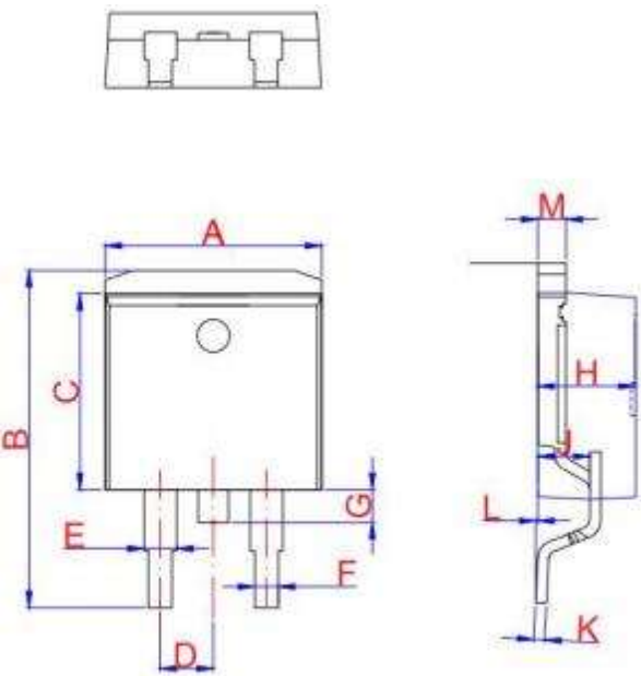
TO-263
