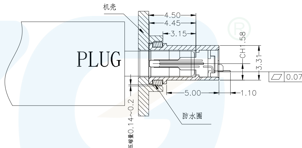
产品防水机构示意图
