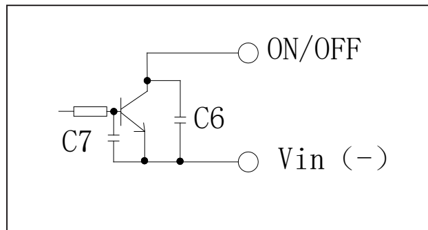
图 C: 晶体管控制方式
