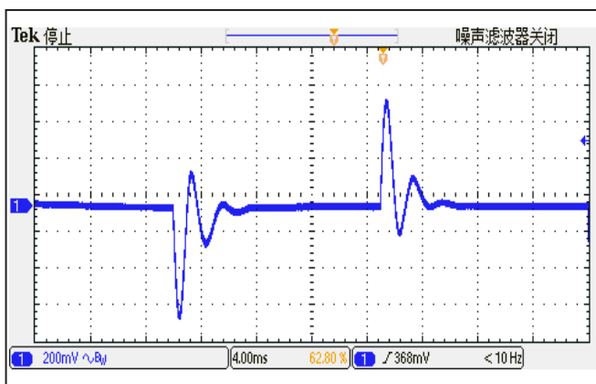
图 4: 负载动态响应, Vin=24V, Io=50%-75%-50%, 2.5A/µs, TC=25°C, CH1: 输出电压
