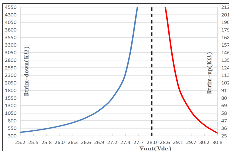
TRIM 电阻 VS 输出电压曲线
