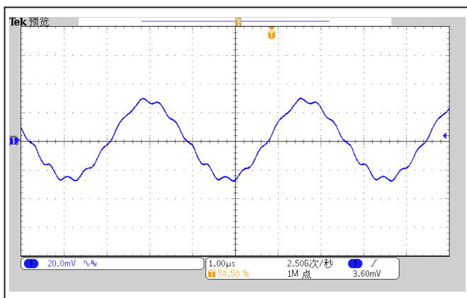
图 3: 输出纹波电压, Vin=24V, Io=2.7A, TC=25°C
