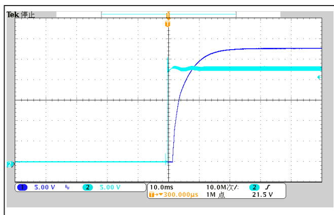
图 5: 启机延时, Vin=24V, Io=2.7A, TC=25°C CH1: 输出电压, CH2: 输入电压
