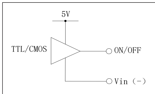
图 E: TTL/CMOS 控制方式
