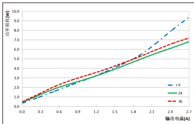
图 2: 功率损耗曲线, TC=25°C
