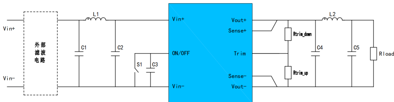
图 A：典型应用电路
